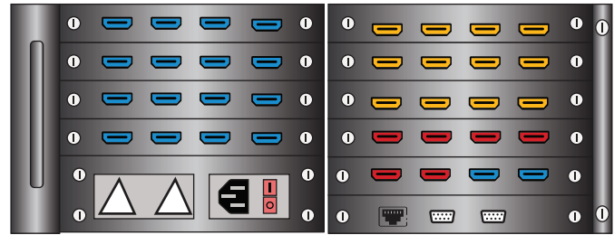
AVW-2418AK : 3U chassis
